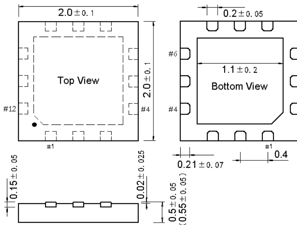
图 4-4 QFN12 封装
