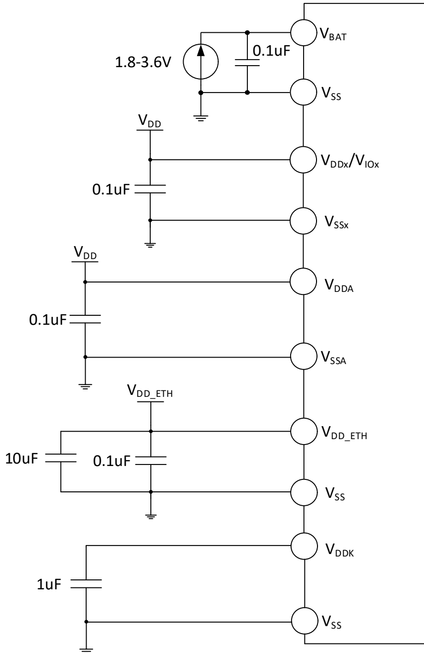
图 4-1-2 CH32V317 常规供电典型电路
