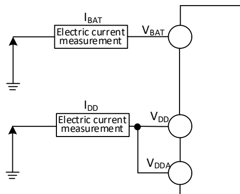
图 4-2-1 GH32V303/305/307 电流消耗测量
