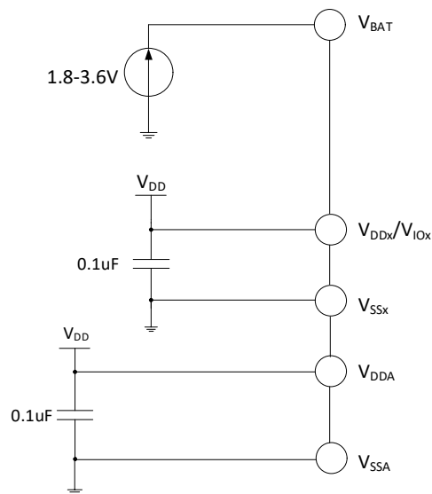
图 4-1 常规供电典型电路
