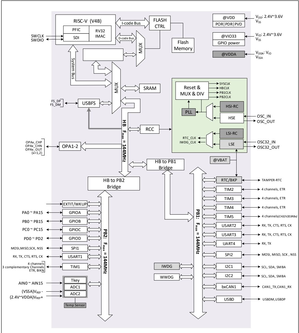
图 2-1 系统框图
